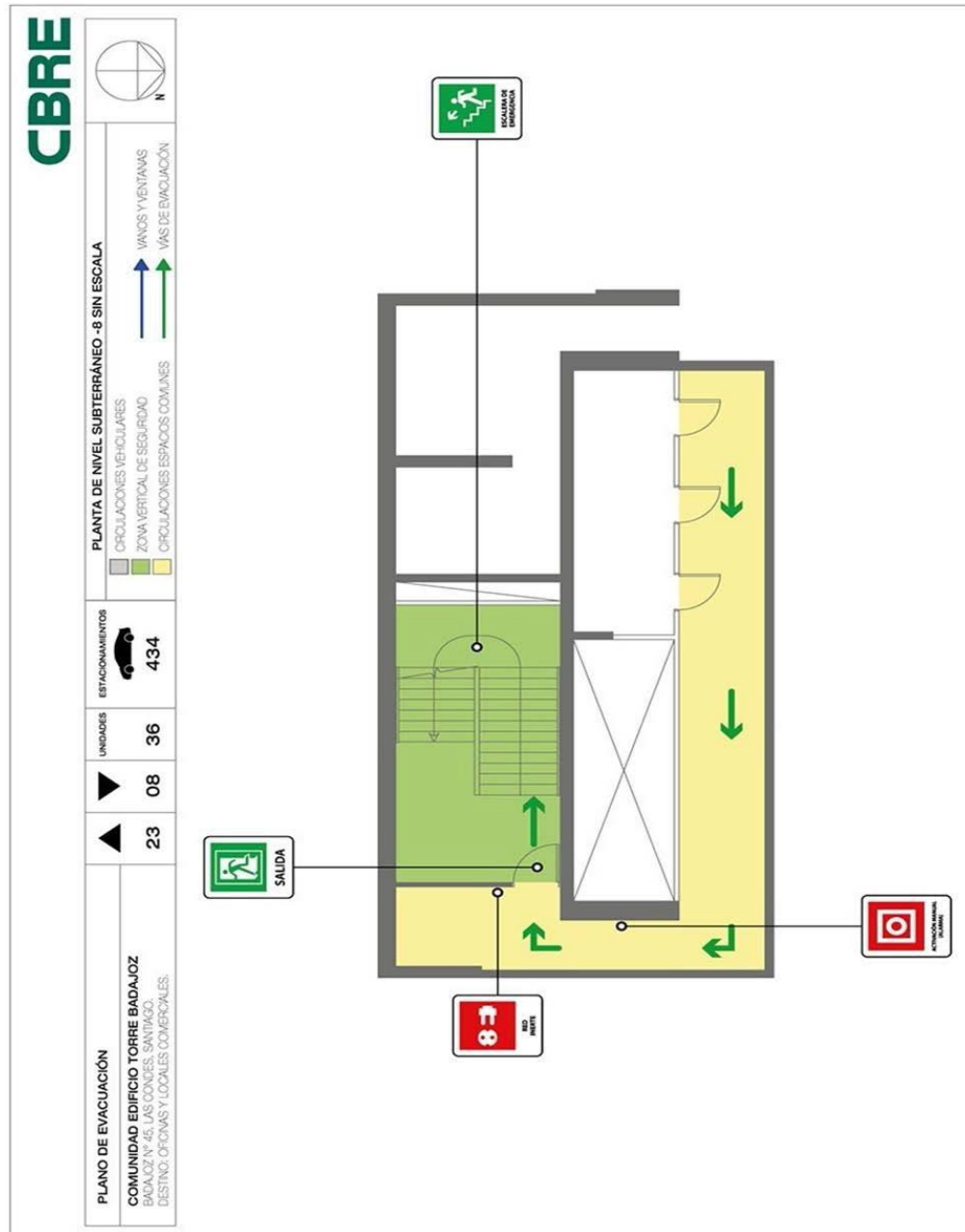
PLANO SUB-8
